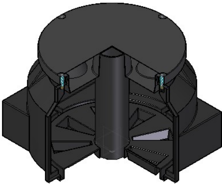
támasztó cső a nagyobb terhelhetőségért
